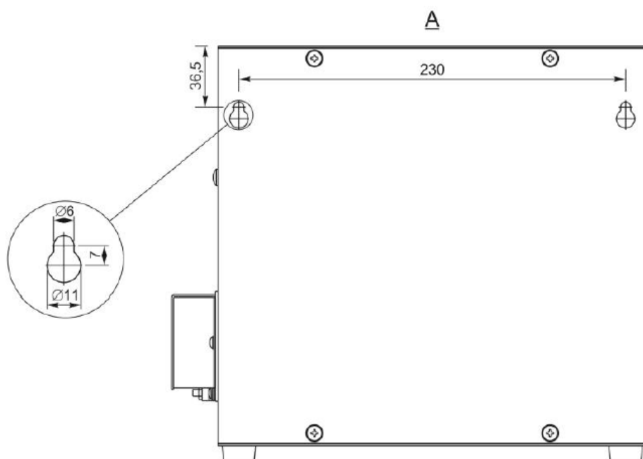
Габаритные и установочные размеры стабилизаторов напряжения переменного тока LIDER PS1200W-30
