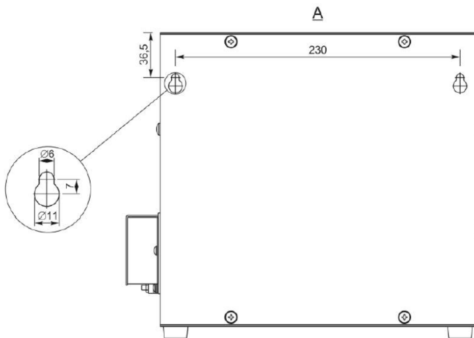
Габаритные и установочные размеры стабилизаторов напряжения переменного тока LIDER PS2000W-30
