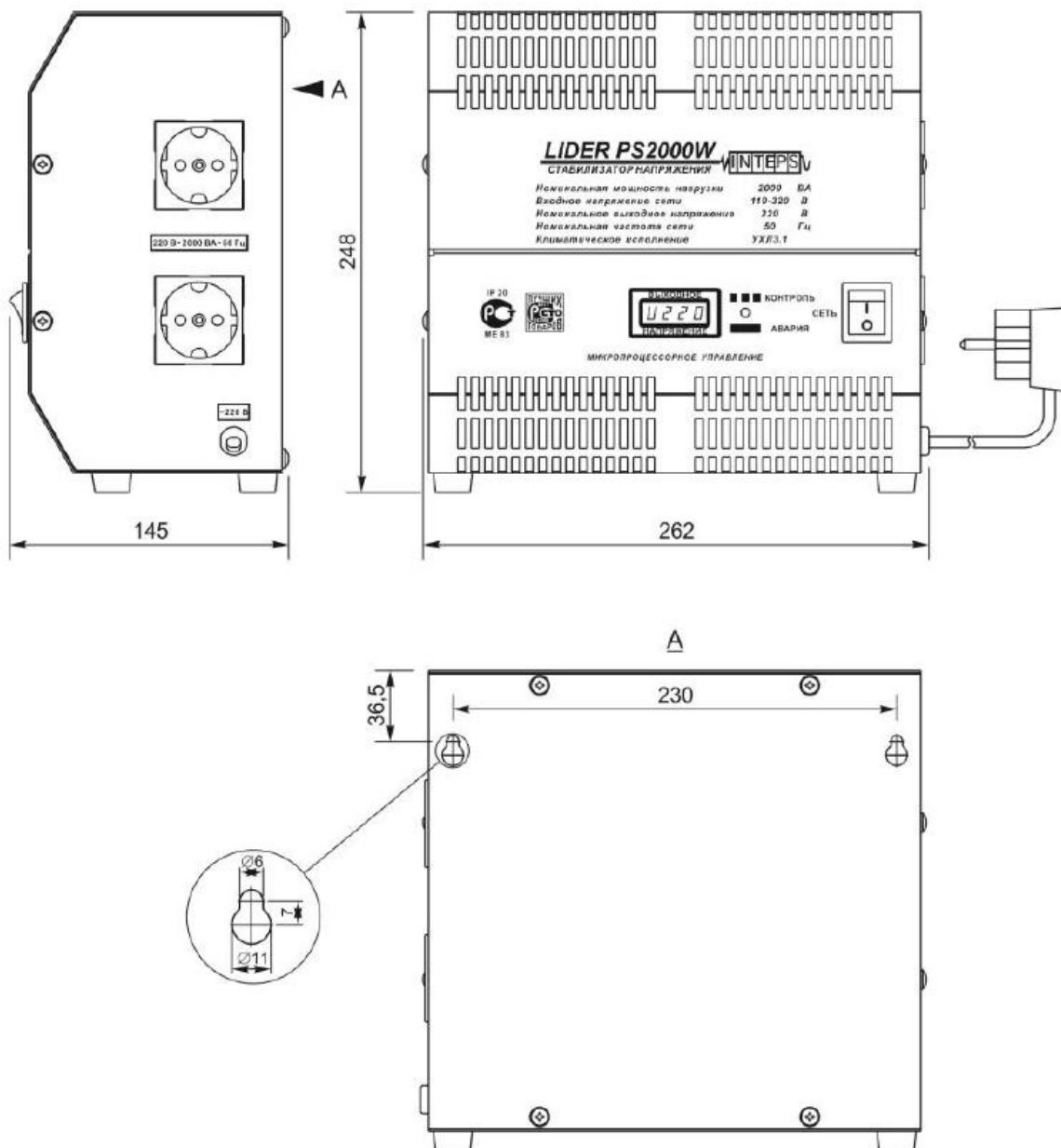
Габаритные и установочные размеры стабилизаторов напряжения переменного тока LIDER PS900W-30
