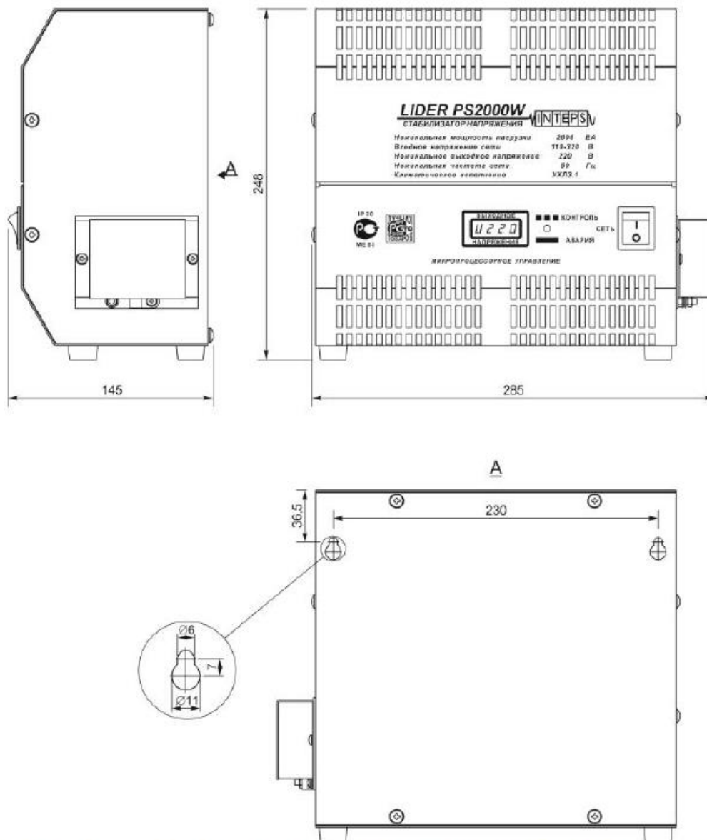
Габаритные и установочные размеры стабилизаторов напряжения переменного тока LIDER PS900W-50
